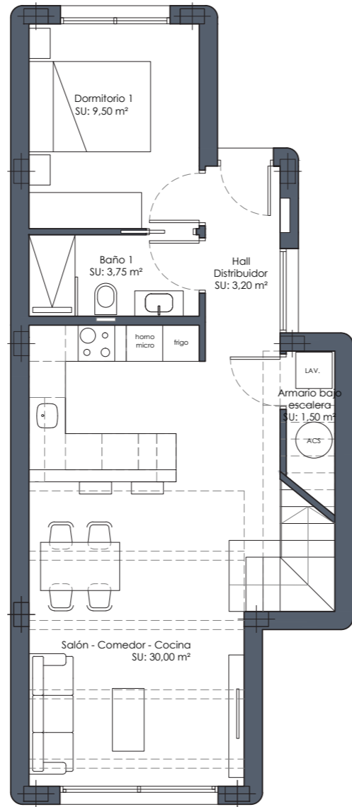
PLANTA BAJA
